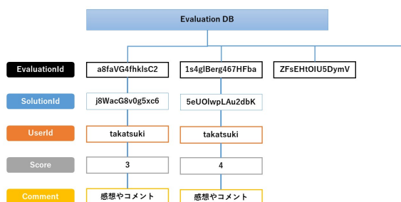
図 4 評価概念モデル
