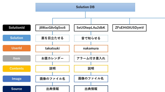
図 3 対処法概念モデル
