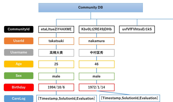
図 5 コミュニティ概念モデル
