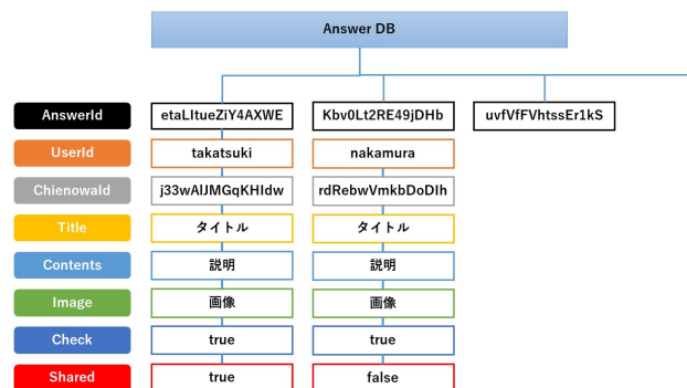
図 7 回答概念モデル
